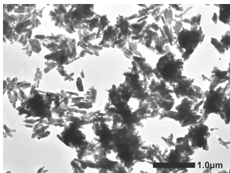
YM1100のTEM画像
