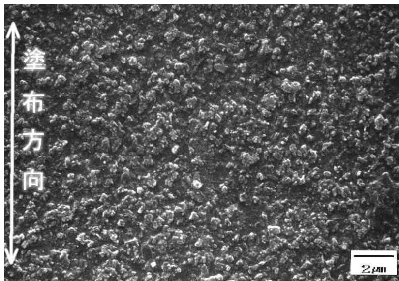
YM1100の塗膜のSEM画像
