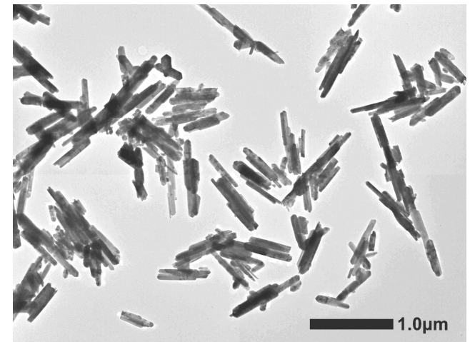
LL-XLOのTEM画像
