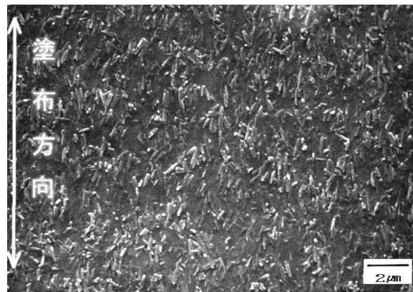
LL-XLOの塗膜のSEM画像
