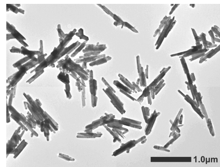
LL-XLOのTEM画像
