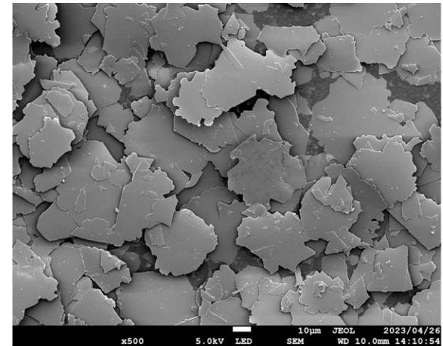
AM-200PのSEM画像
