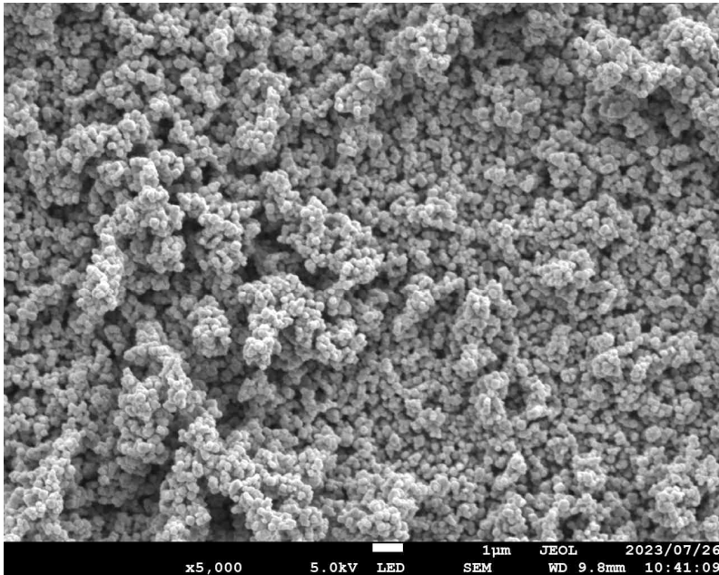
BL-100のSEM画像
