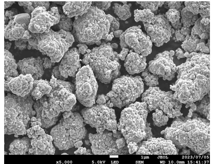
BL-SPのSEM画像
